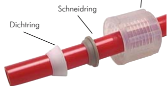
Anschlußprinzip 2
