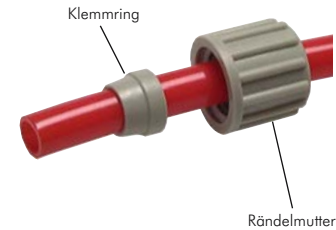
Anschlußprinzip 1
