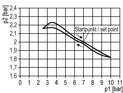
Hysteresse
