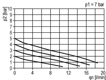
Durchflussdiagramm
