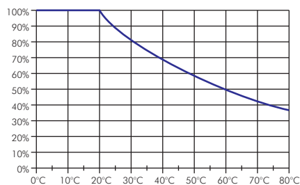
Druck/Temperaturdiagramm PUN-Schläuche
