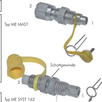
Typ ME SVST 162
