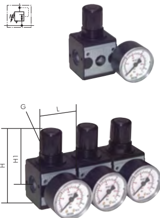
Montagebeispiel für Dreierverkopplung Ausgänge mit verschiedenen Drücken
