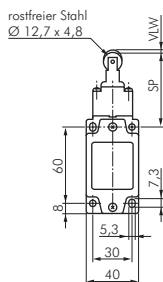
Rollenstößel
