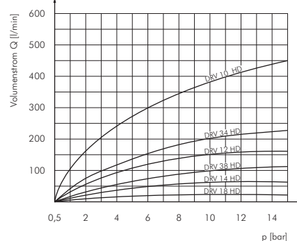
Durchflussrichtung: B-A p Kennlinie freier Durchfluss über Rückschlagventil
