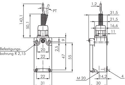
Federstab Edelstahl
