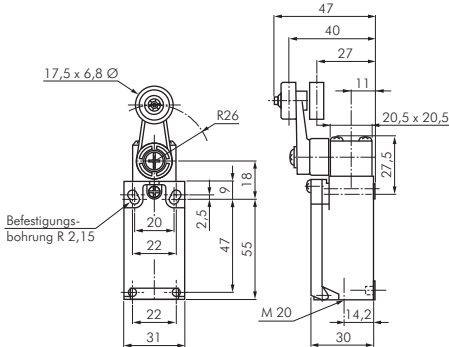
Rollenhebel Kunststoff
