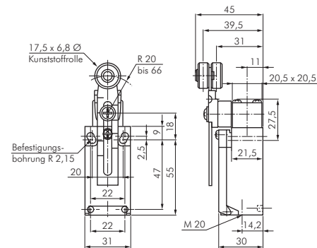
Rollenhebel verstellbar
