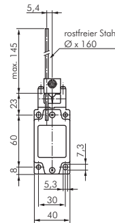
Stangenhebel verstellbar
