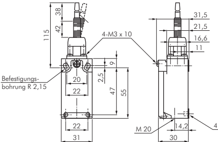
Federstab Kunststoff
