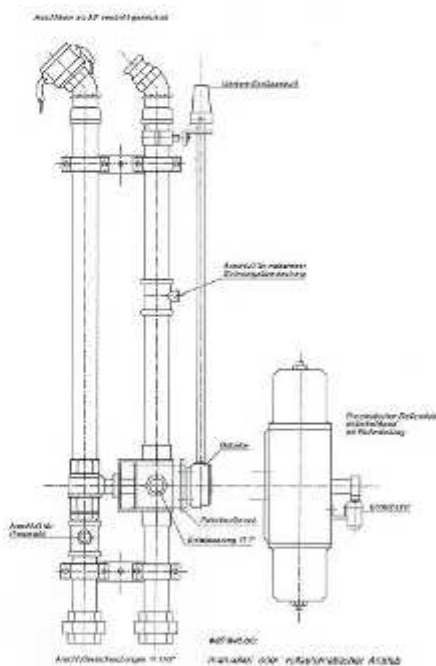
Erster Kombihydrant aus dem Jahre 1995
